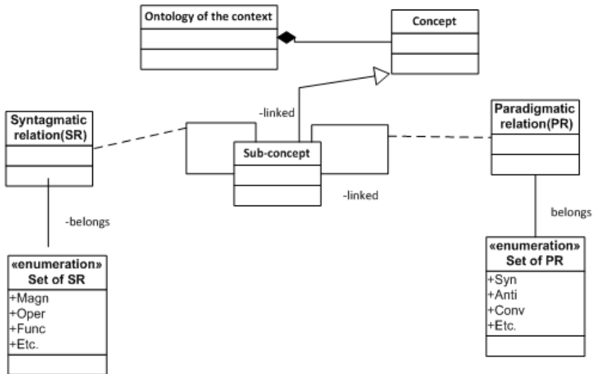
Figure 8 : Méta-modèle de l'ontologie du contexte
