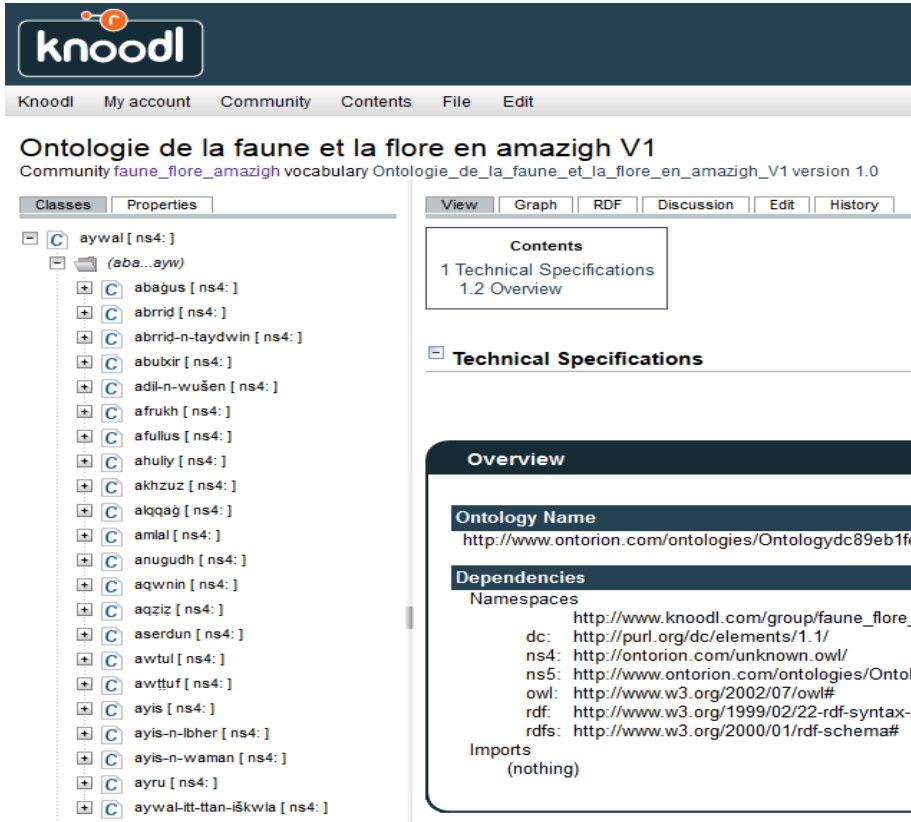
Figure 11: Extrait de l'ontologie à partir du Cloud (Knoodl)
