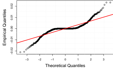
(d) Unconstrained ATOM ZIT. QQ-Plot
